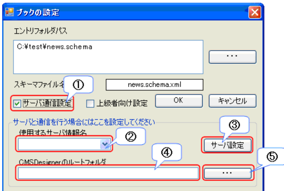
(図 ブックの設定画面 サーバ通信設定パネル表示時)
